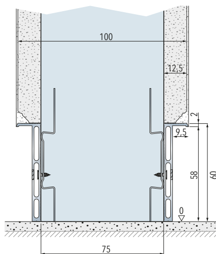
Auf Gipskartonwänden, einlagige Beplankung .
