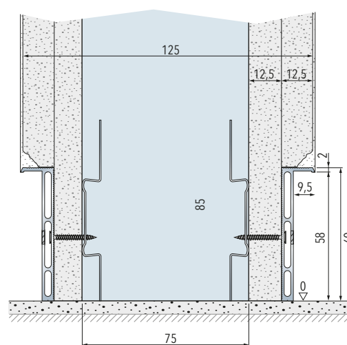
Auf Gipskartonwänden, zweilagige Beplankung .
