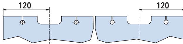
Einsetzbeschlag bis 80 kg (pro Paar)
